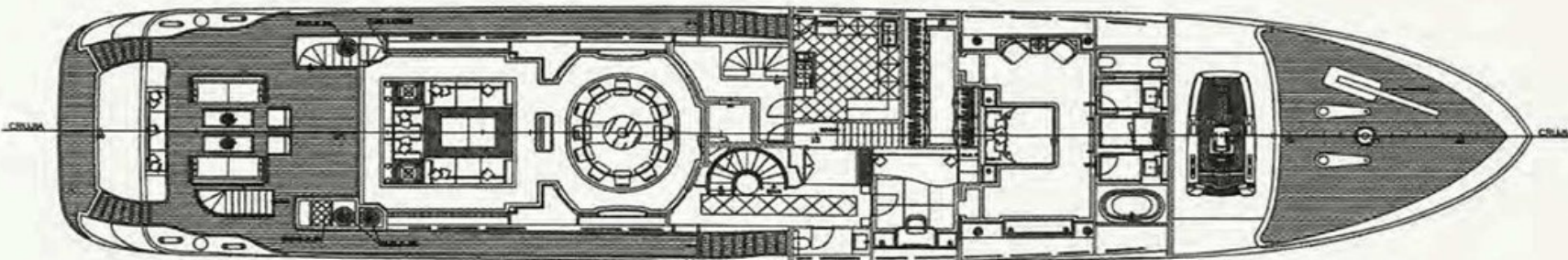
CUBIERTA PRINCIPAL
